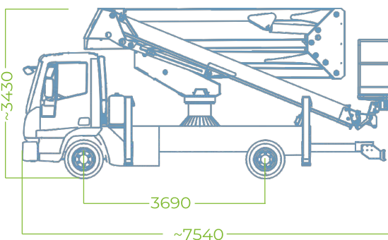
IVECO EUROCARGO
